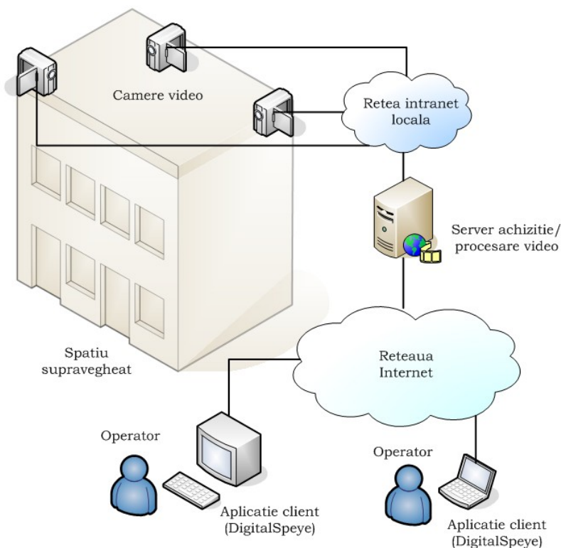
Figura 4-1. Arhitectura generală a sistemului DigitalEye.
